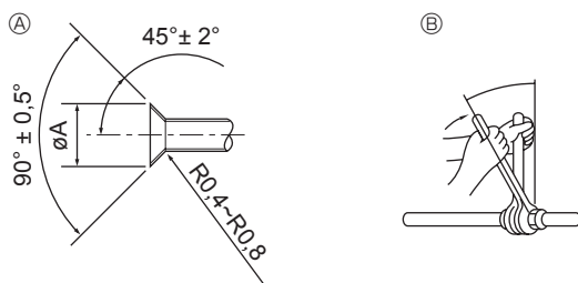
Ⓐ Mått för flänsning Ⓑ Åtdragningsmoment för flänsmutter
