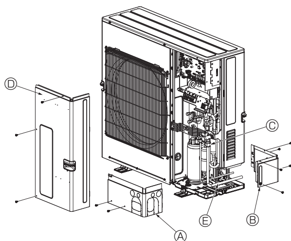
Ⓐ Hölje för främre rörledningsmaterial Ⓑ Hölje för bakre rörledningsmaterial Ⓒ Stoppventil Ⓓ Servicepanel Ⓔ Krökningradie : 100 mm - 150 mm
