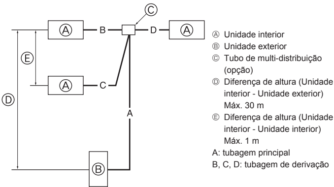
<Limites da instalação da tubagem do refrigerante>
