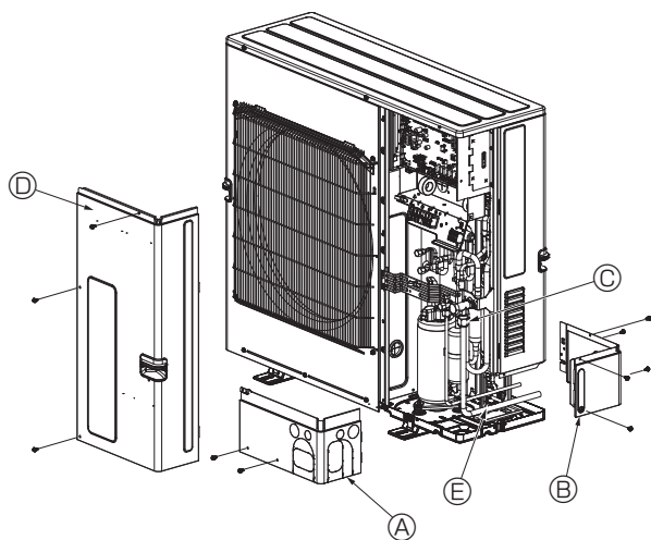
Α Εμπρόσθιο κάλυμμα σωληνώσεων Β Πίσω κάλυμμα σωληνώσεων Γ Βαλβίδα διακοπής Δ Καπάκι εξυπηρέτησης Ε Ακτίνα ζώνης : 100 mm - 150 mm
