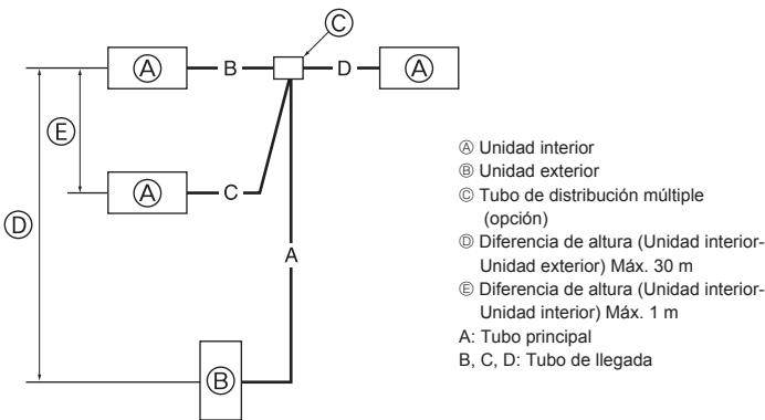
<Límites de la instalación de tubos de refrigeración>
