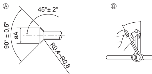
(A) Dimensioni di taglio per raccordo a cartella (B) Coppia di serraggio del dado a cartella
