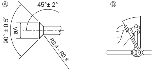
Ⓐ Geçme kesim ölçüleri Ⓑ Geçme somun sıkıştırma torku
