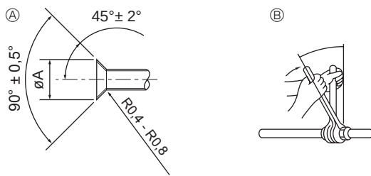
Ⓐ Afsnijmaten tromp Ⓑ Aanhaalmoment flensmoer
