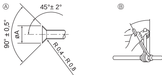
A Rozměry rozšíření B Uťahovací moment převlečné matice
