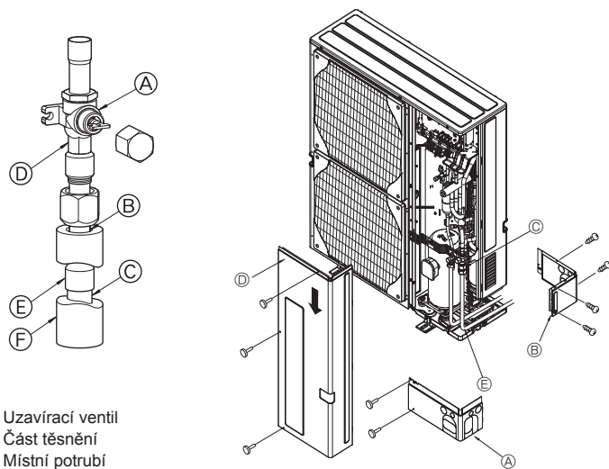
A Přední kryt potrubí B Kryt potrubí C Uzavírací ventil D Servisní panel E Poloměr ohybu: 100 mm – 150 mm
