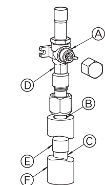
Ⓐ Zawór odcinający Ⓑ Odcinek uszczelniający Ⓒ Lokalna instalacja rurowa Ⓓ Odcinek dokręcany za pomocą 2 kluczy Ⓔ Rura połączeniowa Ⓕ Osłona rur
