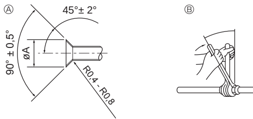
Ⓐ Abmessungen der Aufweitungsanschlüsse Ⓑ Anzugsdrehmoment für die Konusmutter
