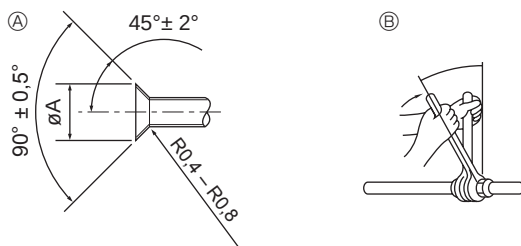
Ⓐ Wymiary przycinania kielichów Ⓑ Moment dokręcania nakrętek kielichowych
