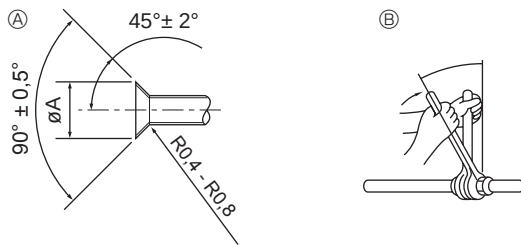
Ⓐ Avarusmitat Ⓑ Kartiomutterin kiristysmomentti
