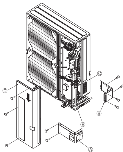
Ⓐ Pijpbedekking aan voorzijde Ⓑ Pijpbedekking Ⓒ Afsluitkraan Ⓓ Onderhoudspaneel Ⓔ Buigstraal : 100 mm - 150 mm
