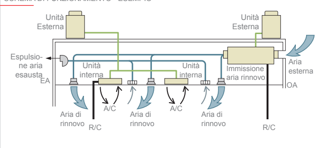
SCHEMA DI FUNZIONAMENTO - ESEMPIO
