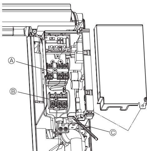
Α Μπλοκ ακροδεκτών τροφοδοσίας ρεύματος (TB2) Β Μπλοκ ακροδεκτών μεταφοράς (TB5) Γ Σφιγκτήρας καλωδίων
