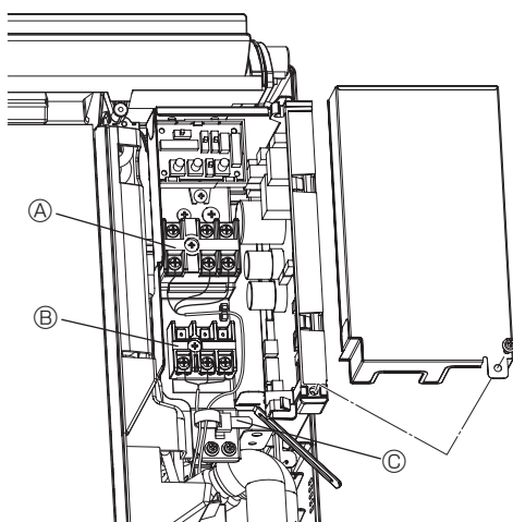
A Bloque de terminales de la fuente de alimentación (TB2) B Bloque de terminales de la transmisión (TB5) C Prensaestopas
