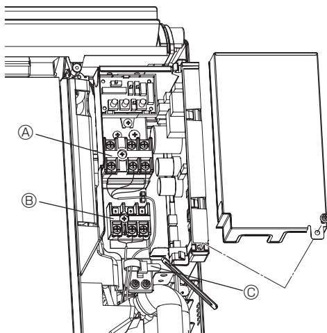
Ⓐ Blocco terminale di alimentazione (TB2) Ⓑ Blocco terminale di trasmissione (TB5) Ⓒ Serracavo
